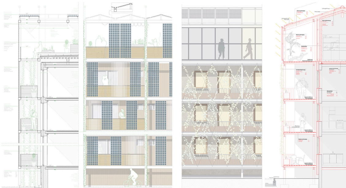
Fig. 16: Eva Grotter and Marie Christine Häußler, section 1:20 / Fig. 17: Julia Hager and Daniel Jäger, section 1:20
